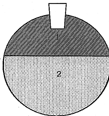
図5 玉切りの手順とくさびの位置
